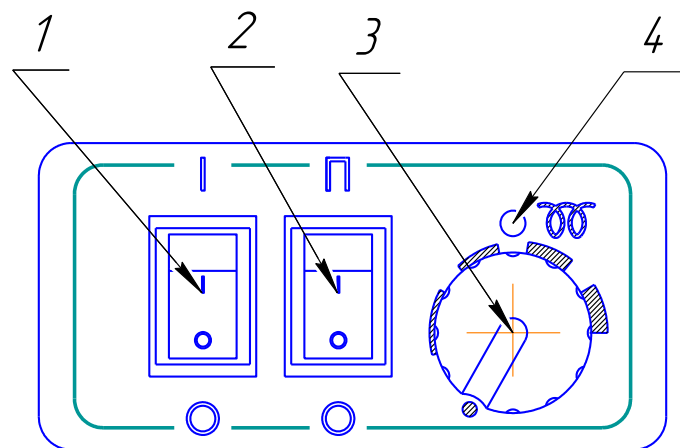
Рис. 3 – Лицевая панель пульта ПУ- 7М
